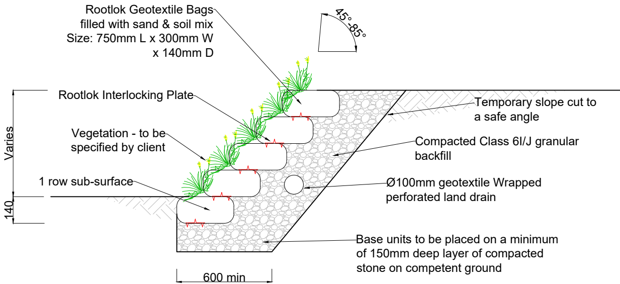
Gravity Wall 45° Batter
