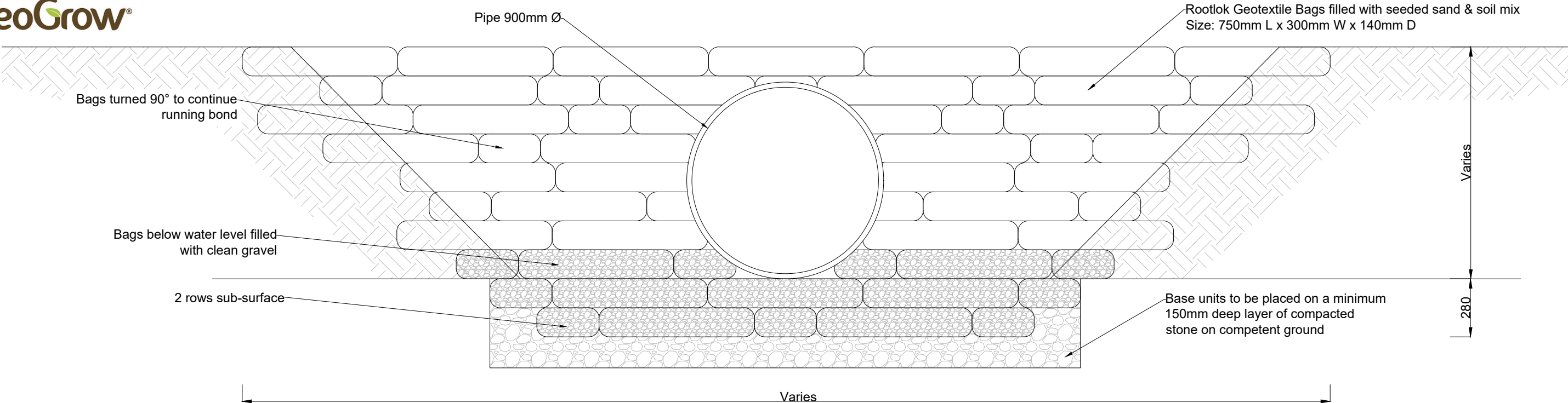
Elevation
