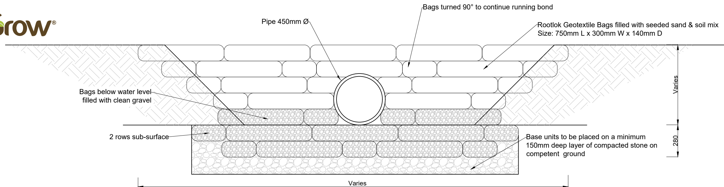
Elevation
