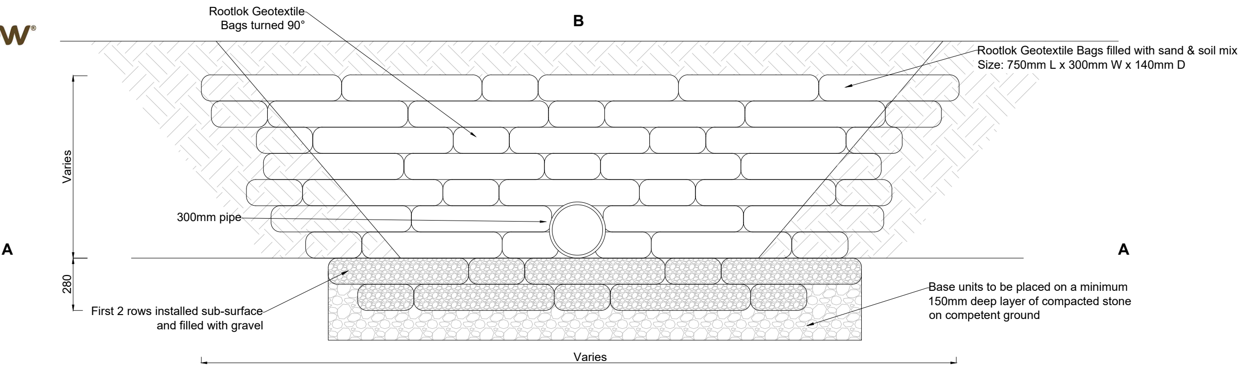
Elevation
